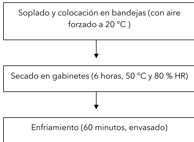
Figura 8. Flujo tecnológico para la elaboración de pastas alimenticias utilizando granular durum - almidón de banano.
