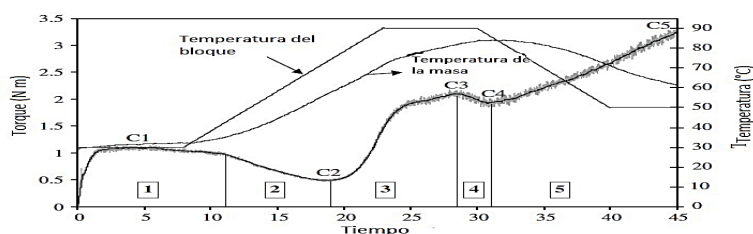
Figura 7. Curva típica registrada en el Mixolab® empleando el protocolo propuesto por Chopin Technologies.
