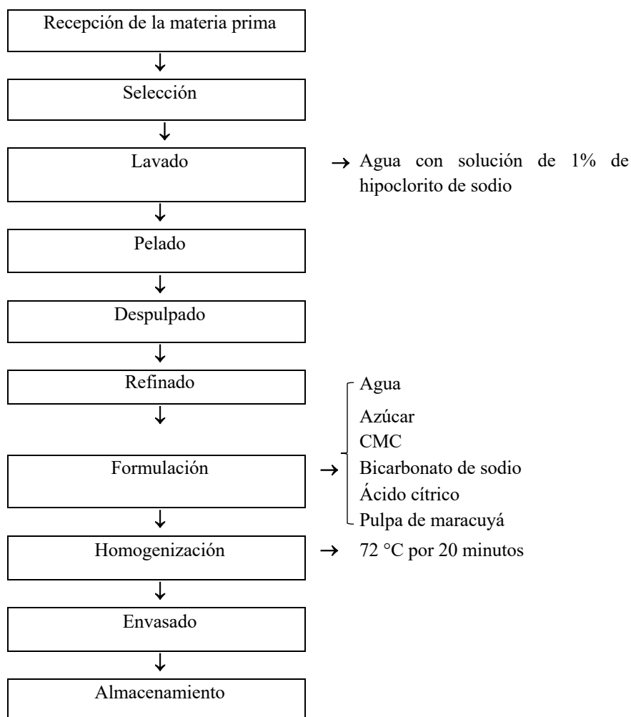
Ilustración 12: Diagrama de flujo para la elaboración de jarabe de maracuyá
