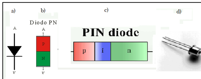
Figura 1. a) Símbolo del diodo, b) Composición de un diodo unión PN, donde P (silicio extrínseco tipo P) y N (silicio extrínseco tipo N), c) Composición de un diodo unión PIN, donde P (silicio extrínseco tipo P), I (material intrínseco) y N (silicio extrínseco t)
