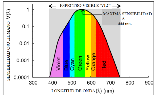
Figura 6. Función luminosidad
