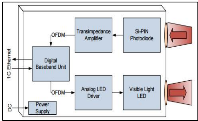
Figura 15. Arquitectura interna de un Transceptor Dongle
