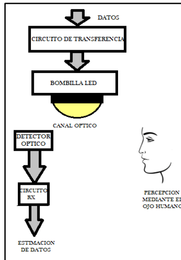
Figura 5. Debido a la doble funcionalidad de VLC, uno debe considerar tanto el detector óptico como el ojo humano. El detector óptico seguido por el circuito del receptor estima los datos transmitidos, mientras que el sistema visual humano construye una imagen, necesariamente percibiendo el color y el brillo de la luz incidente.
