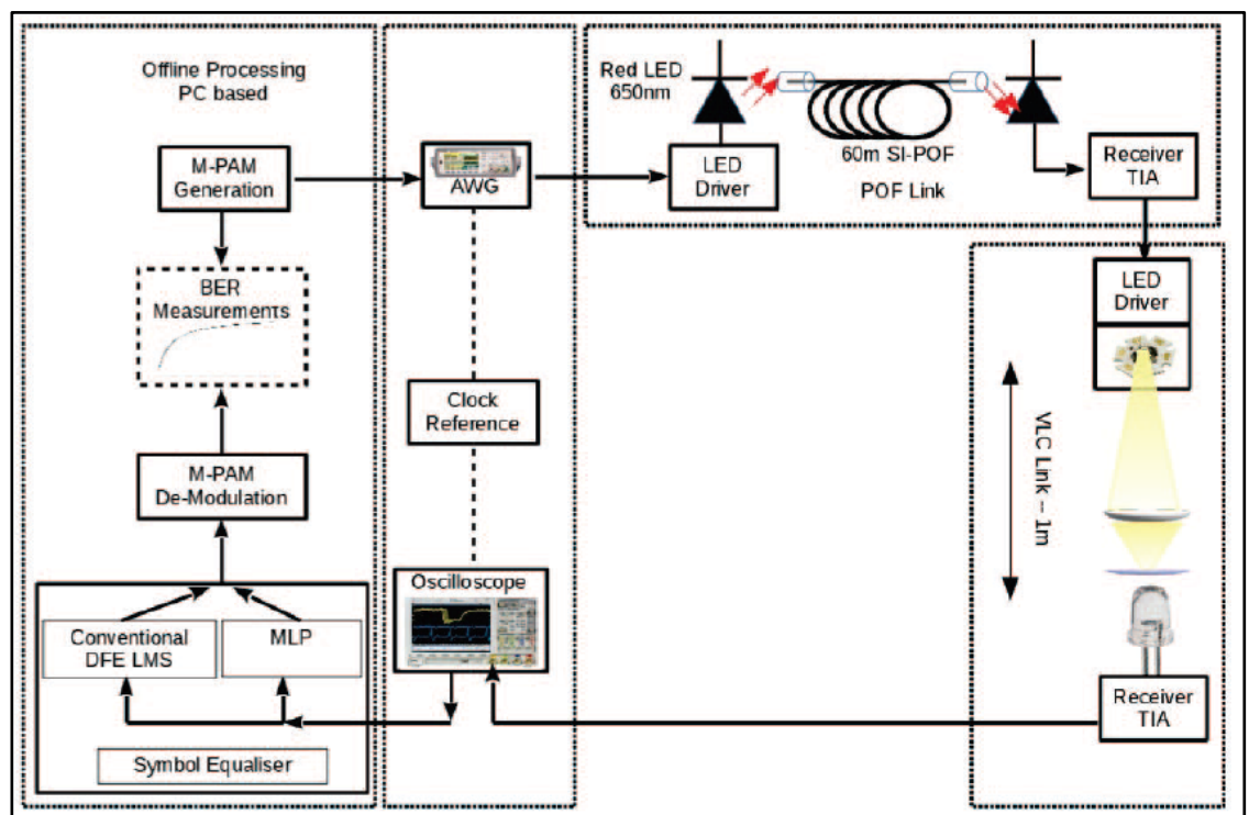
Figura 21. Diagrama de bloques de la configuración experimental para el sistema POF-VLC
