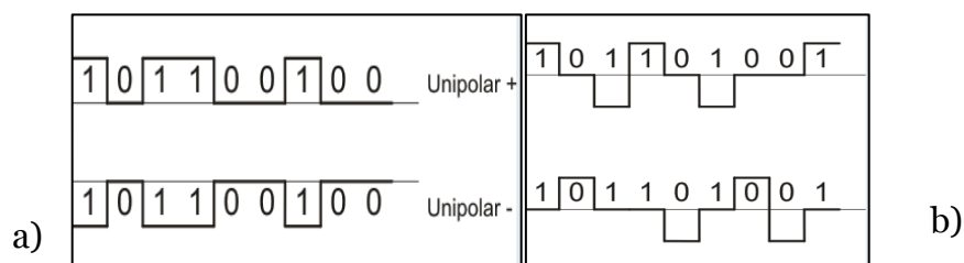
Figura 4. a) Señal Unipolar y b) Señal Bipolar
