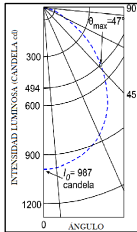
Figura 8. Distribución de la intensidad luminosa.
