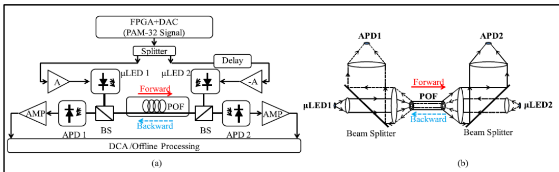
Figura 20. a) Configuración experimental para implementar el enlace BiDi SI-POF; b) esquema de acoplamiento óptico en cada extremo de POF
