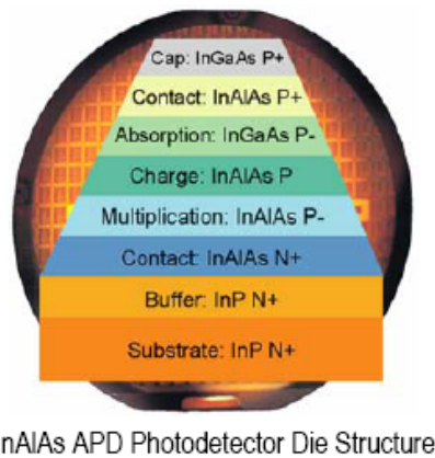
Figura 2. Estructura del fotodetector avalancha APD, del fabricante SPECTROLAB, composición química InAlAs (arseniuro de aluminio-indio o arseniuro de aluminio y aluminio “Aluminium indium arsenide”).
