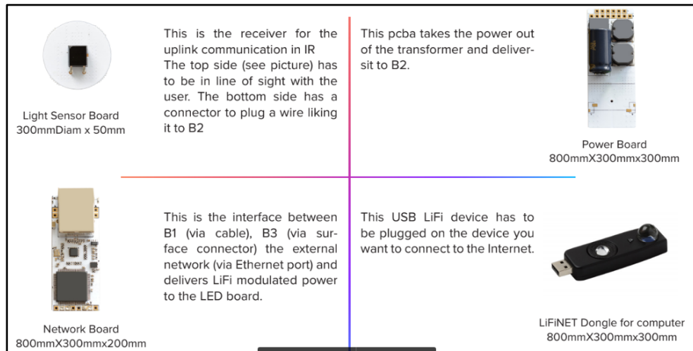
Figura 13. Componentes y descriptiva del modem: Como se puede observar en el lado izquierdo de la parte superior de la figura, este es el receptor que permite la comunicación de enlace ascendente en IR. Tiene que estar en línea de vista con el usuario. En la parte superior derecha de la figura se indica el conector, este PCBA elimina la energía del transformador y la entrega a B2. En la parte inferior izquierda de la figura esta la interfaz entre B1 (por cable), B3 (a través del sur-conector) y el externo de la red (a través del puerto Ethernet) que brinda potencia modulada LiFi a la placa LED. En la parte inferior derecha se muestra el Dongle, este dispositivo USB LiFi tiene que estar conectado en el dispositivo que quiere conectarse a internet.
