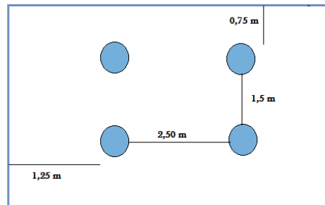
Figura 29. Esquema de planificación de la distribución de las luminarias
