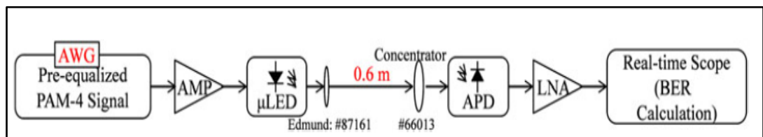
Figura 19. Configuración experimental del VLC utilizando pre-ecualización
