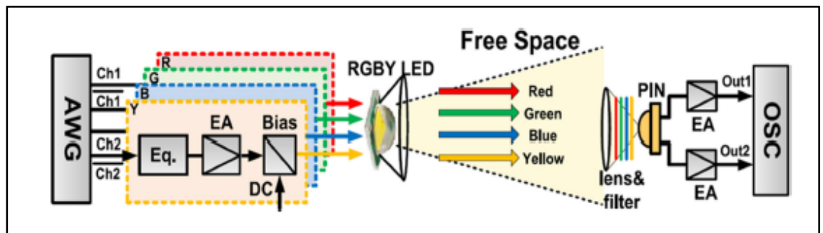
Figura 18. Sistema VLC de cuatro colores de 8 Gbit/s que usa modulación CAP
