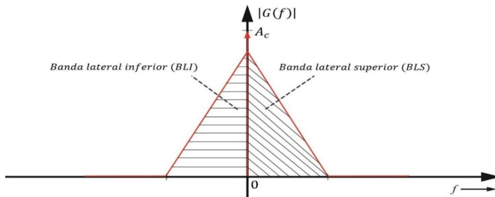
a) Envlovente compleja de una se1al de AM.
