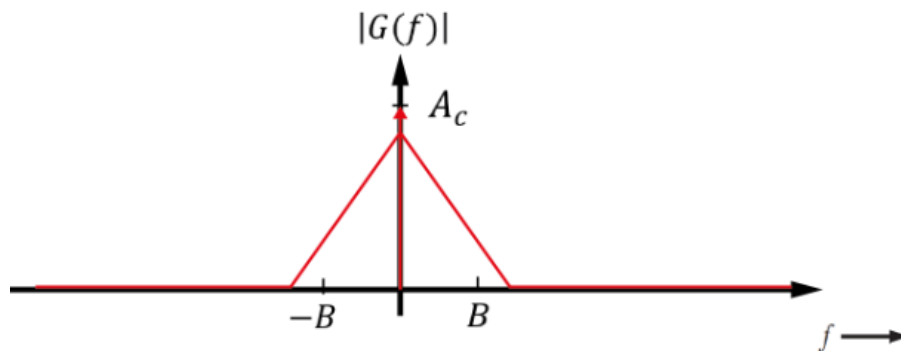
(b) Espectro de la envolvente compleja para una señal AM.
