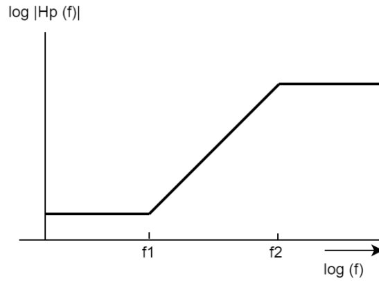
Figura 3.20: Gráfico de Bode de la respuesta en frecuencia de preénfasis
