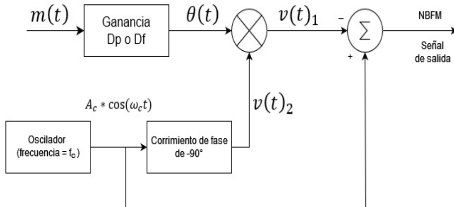
Figura 3.10: Generación de NBFM utilizando un modulador simétrico para FM.
