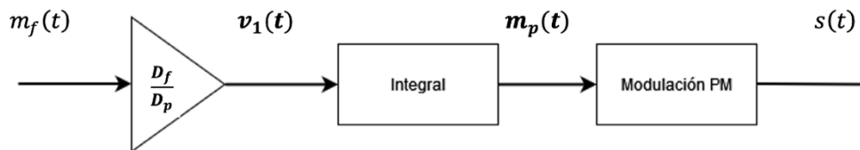
Figura 3.2: Generación de FM utilizando modulador de fase
