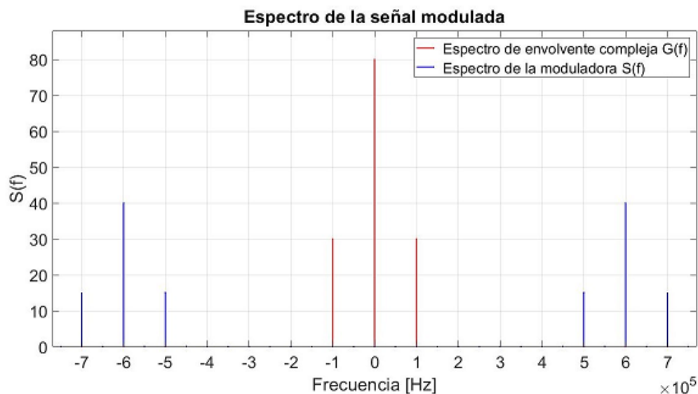
Figura 2.6: Espectro de la señal modulada AM, y envoltura compleja del ejemplo 2.1.
