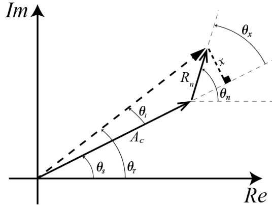
Figura 3.9: Diagrama vectorial para modulación por ángulo, \left(\frac{S}{N}\right)_{in} \gg 1 .
