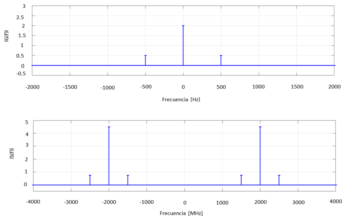
Figura 1. 7: Espectro modulada de una señal AM.
