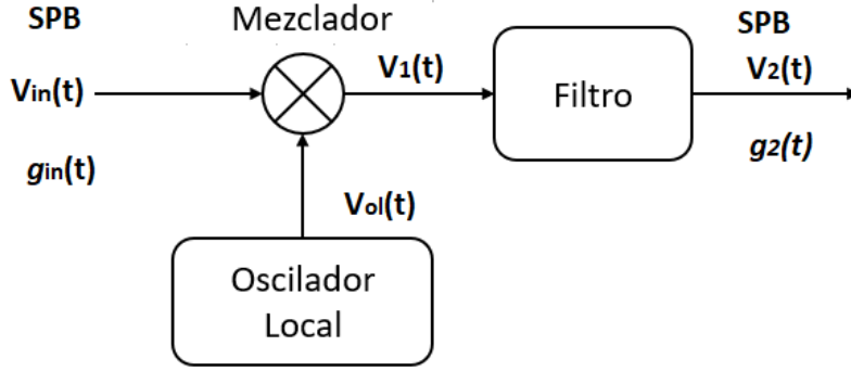
Figura 1. 20: Un mezclador seguido por un filtro para un convertidor elevador o reductor.
