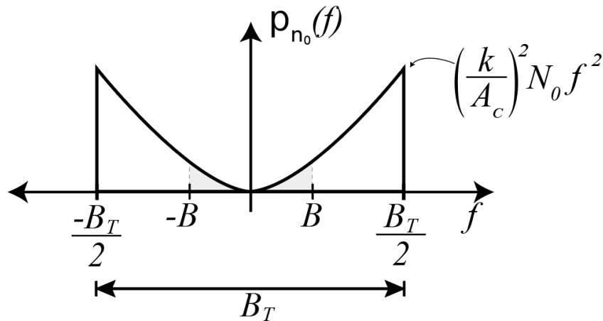
Figura 3.13: DSP para el ruido a la salida del detector para el receptor de señal modulada en FM.
