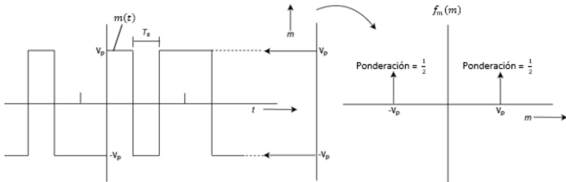
(a) Forma de onda rectangular moduladora (con 1 y 0 binarios igualmente probables)
