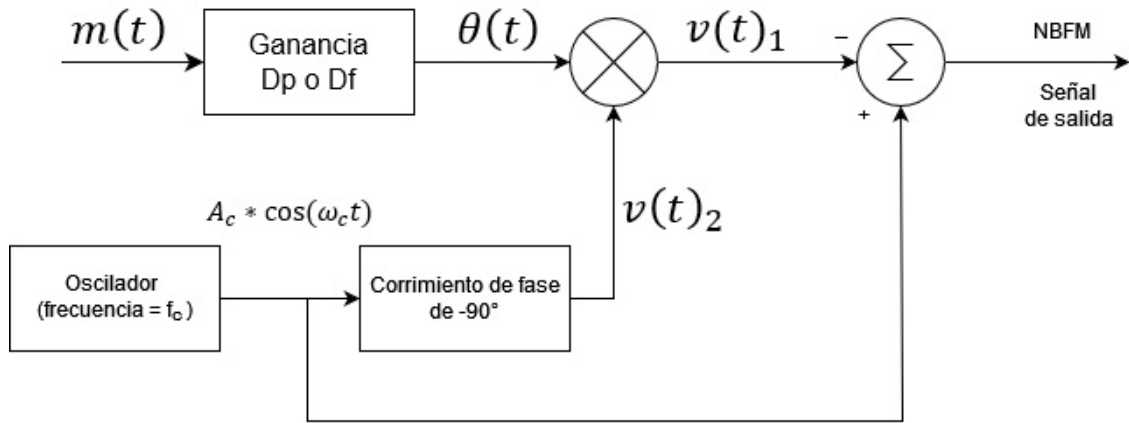
Figura 3.9: Generación de NBFM utilizando un modulador simétrico.
