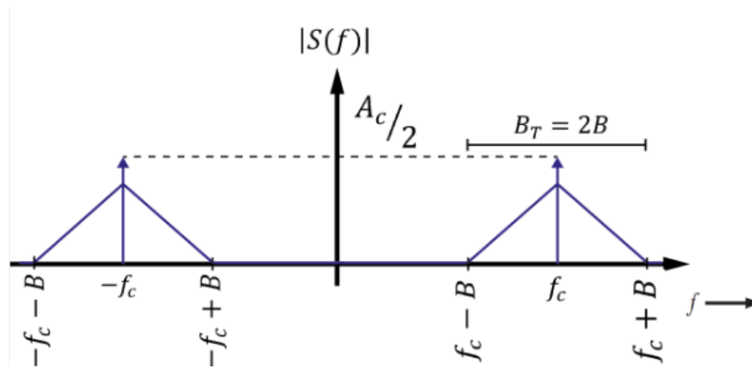
(c) Espectro de una señal AM.
