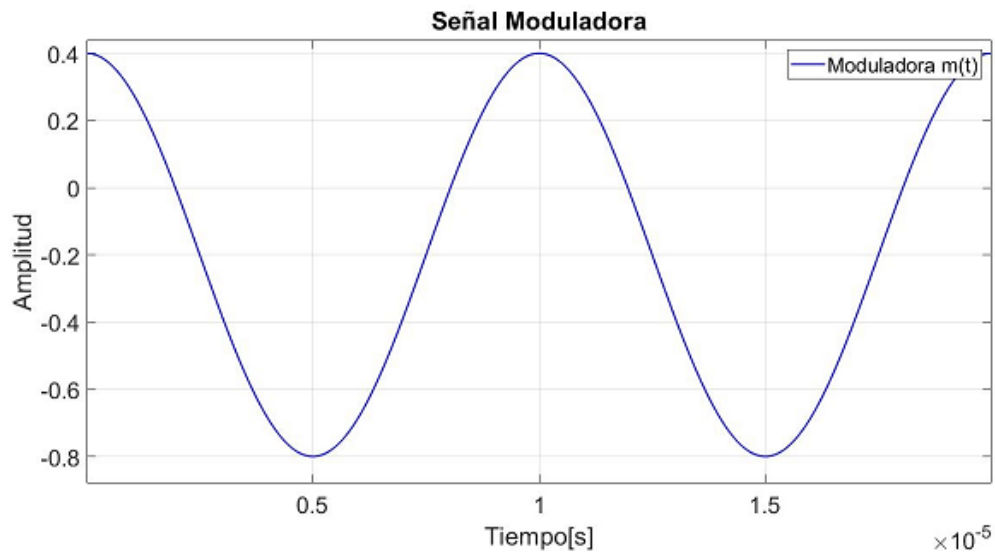
a) Señal moduladora m(t)
