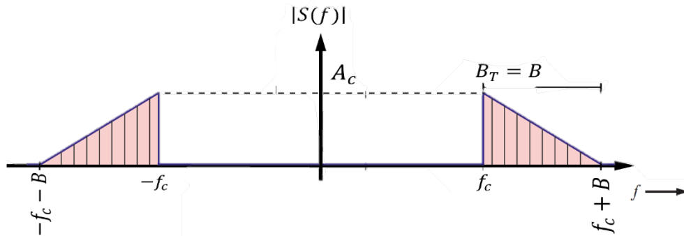
(b) Espectro de la señal modulada USSB
