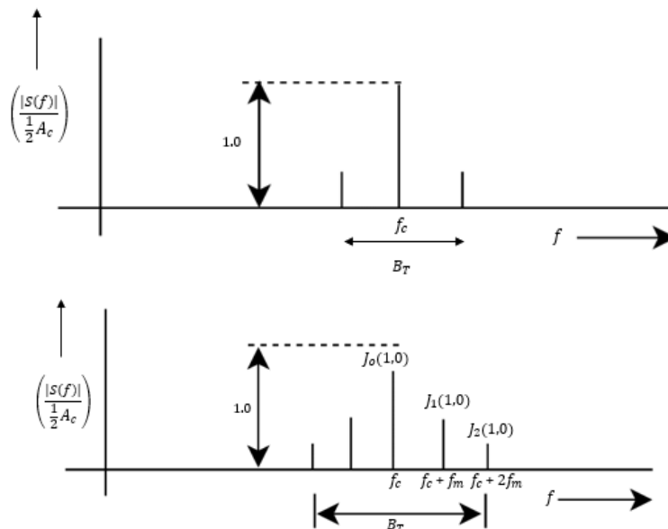
Figura 3.17: Espectros de magnitud para FM o PM con modulación senoidal para índices de modulación 1.0 y 2.0 respectivamente.
