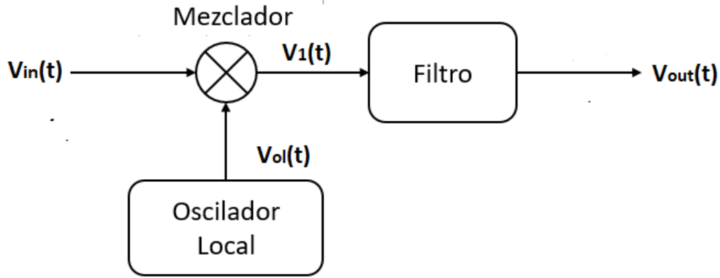
Figura 1. 28: Detector de producto.
