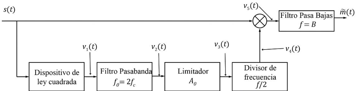
Figura 2.10: Diagrama de bloques para un lazo cuadrático.
