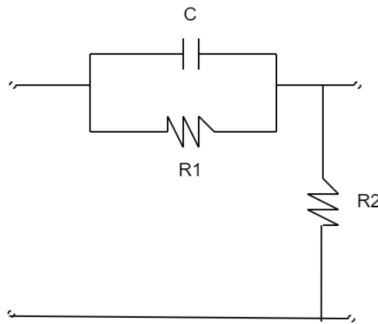
Figura 3.21: Filtro de preénfasis
