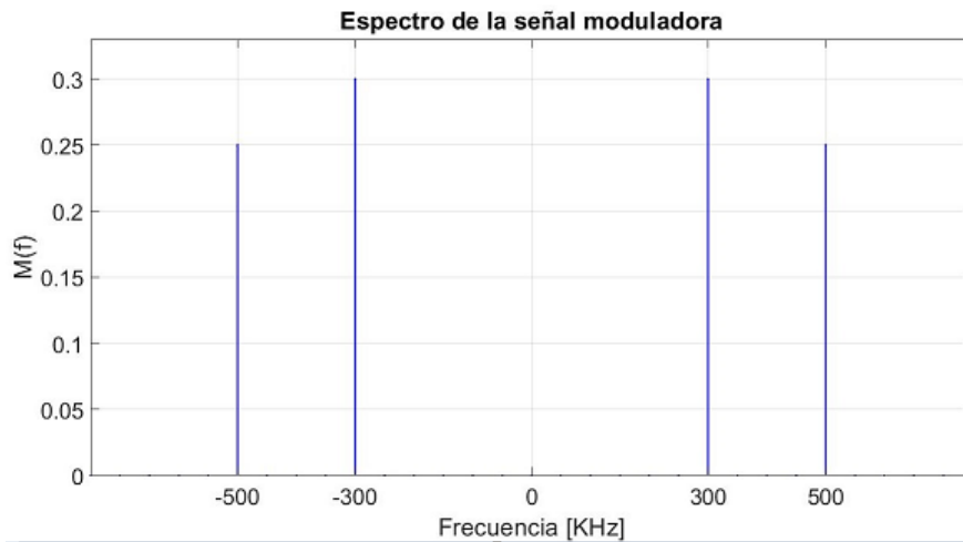
Figura 2.20: Forma de espectro de la señal moduladora del ejemplo 2.3.
