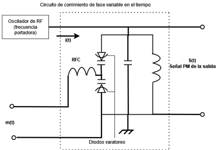
Figura 3.4: Un circuito modulador de fase
