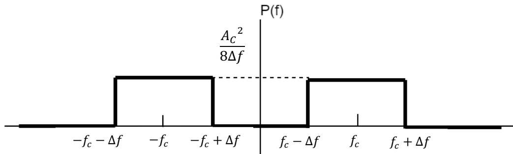
Figura 3.16: PSD de la señal WBFM con modulación triangular, \Delta F = \frac{D_f V_p}{2\pi}
