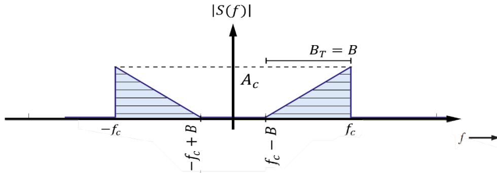
(a) Espectro de la señal modulada LSSB
