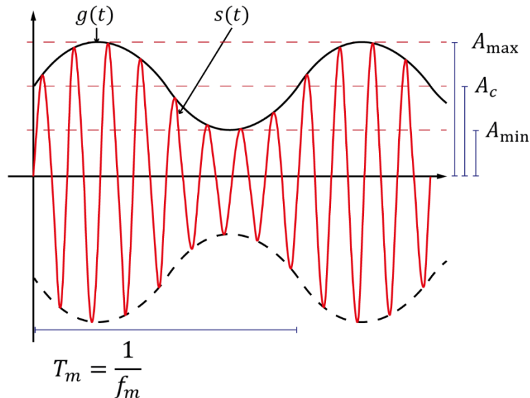
Figura 2.2: Señal modulada y envolvente compleja para AM
