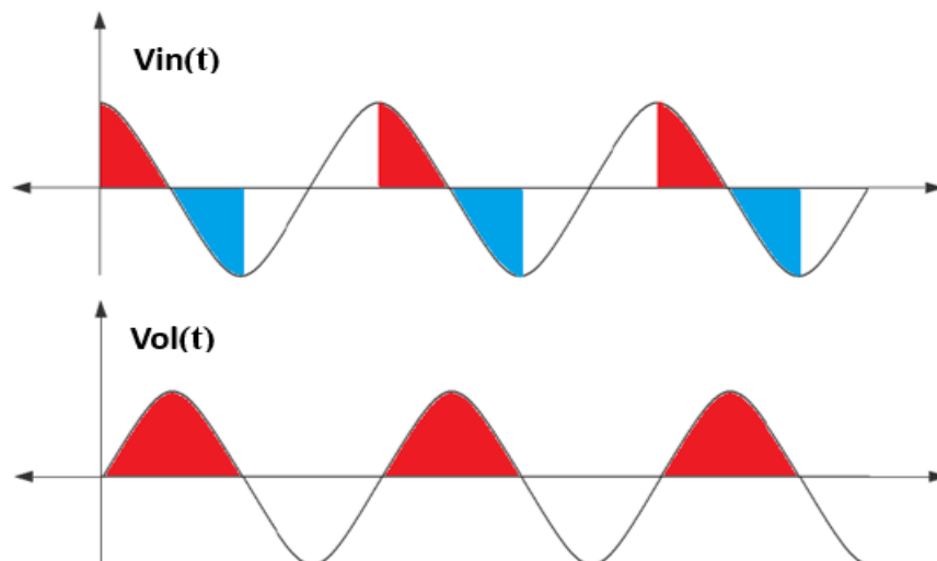
Figura 1. 25: Modulador de 2 cuadrantes.
