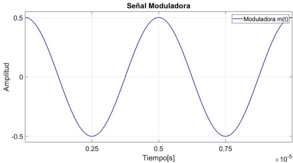
(a) Señal moduladora m(t) del ejemplo 2.2
