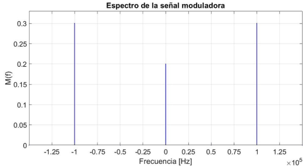
Figura 2.5: Espectro de la señal moduladora.
