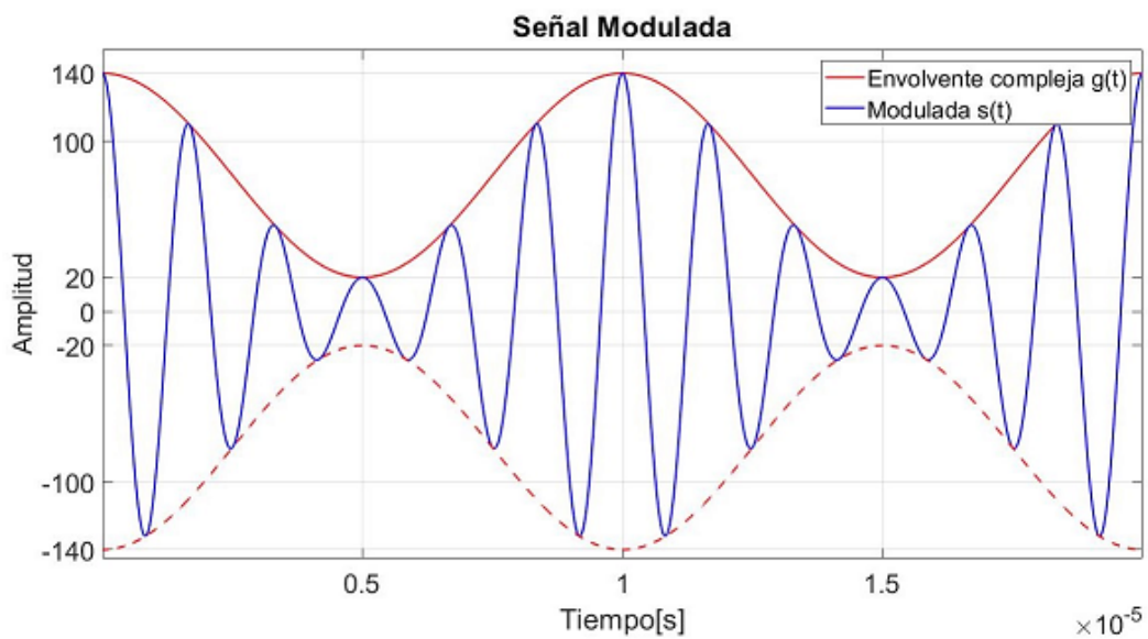
b) Señal modulada s(t) y envolvente compleja real g(t)
