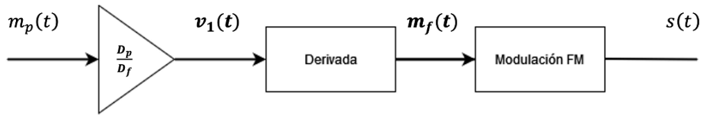
Figura 3.3: Generación de PM utilizando un modulador de frecuencia
