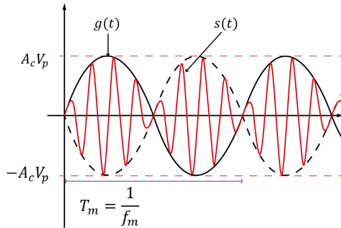
Figura 2.7: Señal modulada y envolvente compleja para DSB-SC
