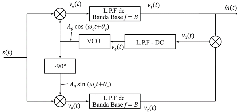
Figura 2.9: Diagrama de bloques para un lazo de costas.
