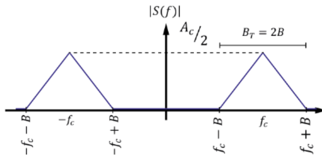
(c) Espectro de una señal DSB-SC.
