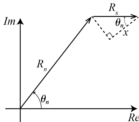
Figura 3.7: Análisis del diagrama fasorial.
