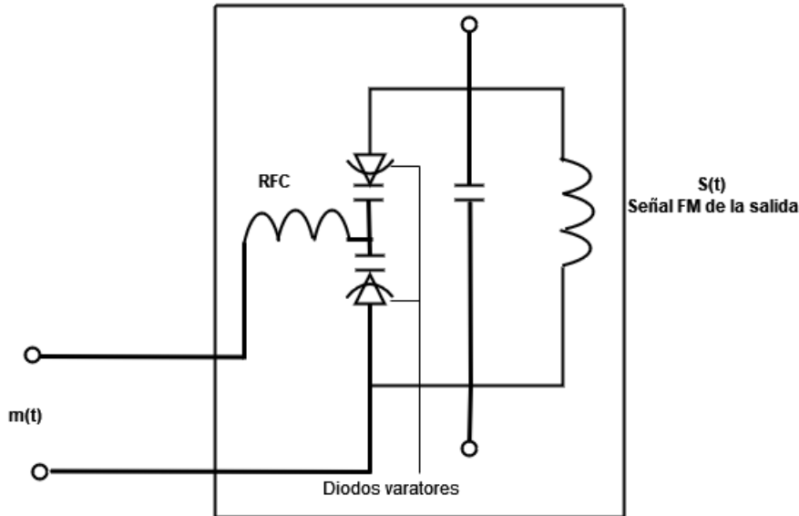
Figura 3.5: Un circuito modulador de frecuencia
