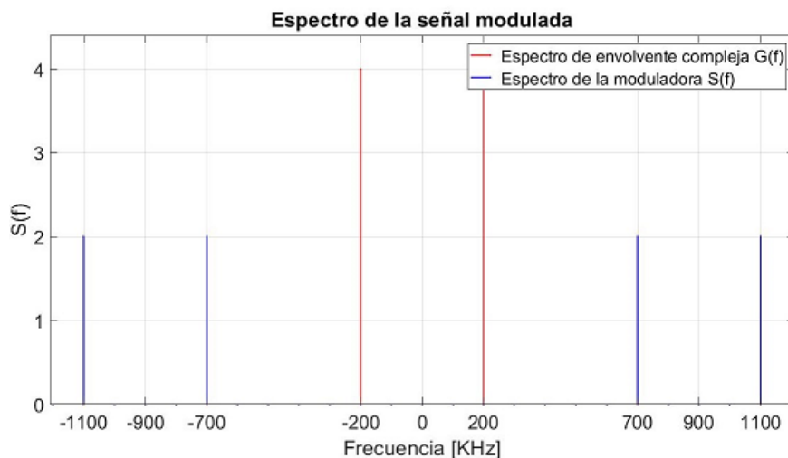
Figura 2.13: Espectro de la envolvente compleja, y señal AM resultante del ejemplo 2.3
