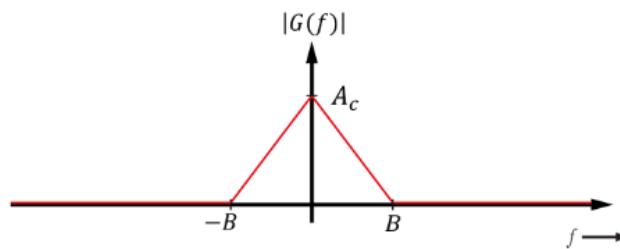
(b) Espectro de la envolvente compleja para una señal DSB-SC.
