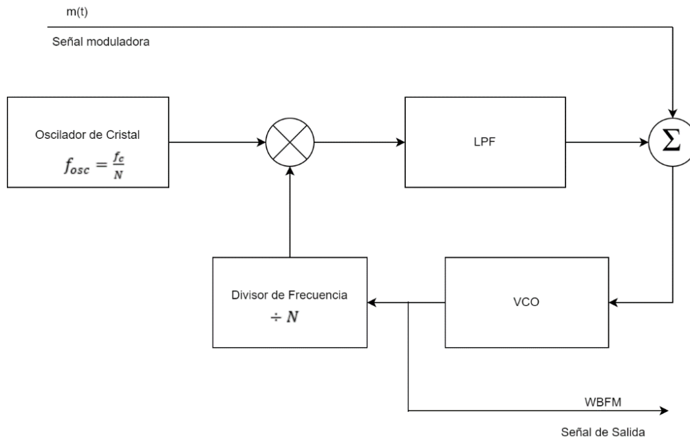
Figura 3.13: Método directo para la generación de WBFM
