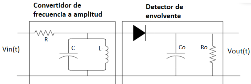
Figura 1. 30: Diagrama de circuito de un detector de pendiente.
