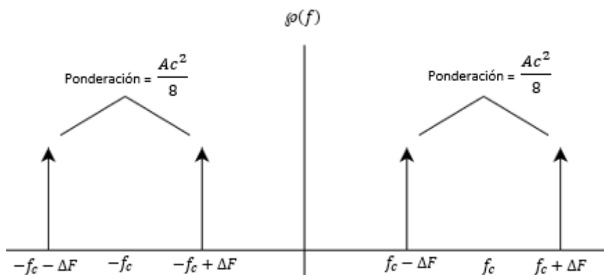
(c) PDF de la FSK de banda ancha con modulación binaria \Delta F = D_f V_p / 2\pi
