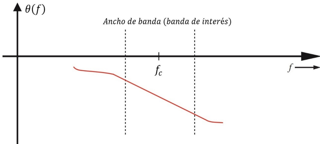
Figura 1. 10: Respuesta de fase de un canal pasabanda sin distorsión.
