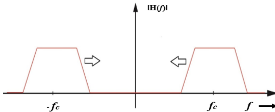
b) Respuesta típica de filtro pasabanda.
