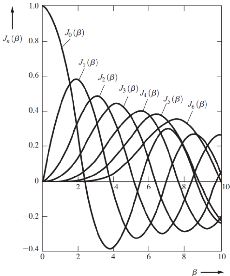
Figura 3.8: Funciones de Bessel para n=0 a n=6
