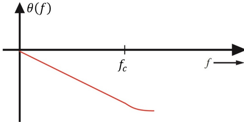
Figura 1. 14: Respuesta común de la fase de un filtro Bessel.
