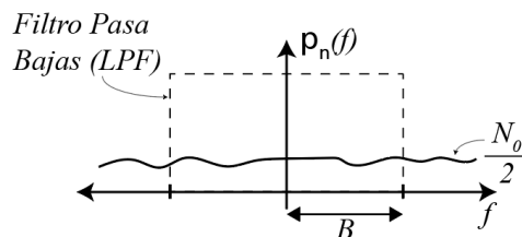
Figura 3.3: DSP del ruido en sistema banda base.
