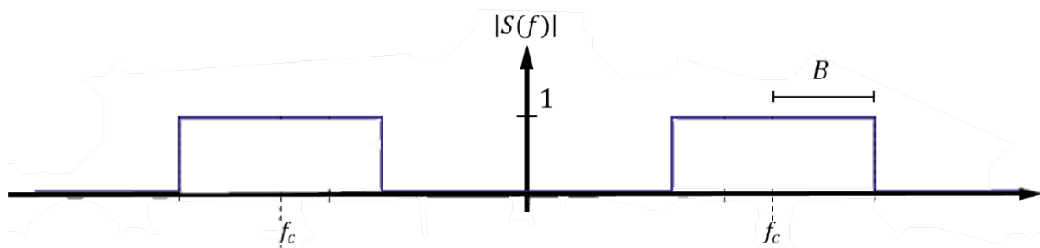
(b) Señal DSB-SC
