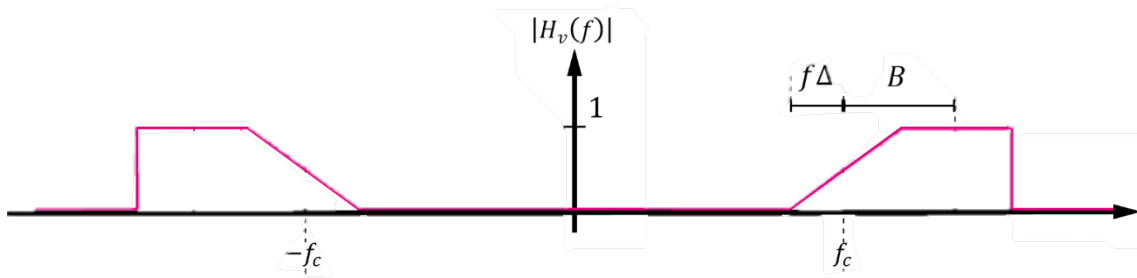
(c) Respuesta de Filtro de Banda Vestigial
