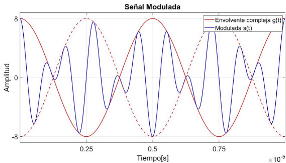
(b) Señal modulada s(t) y envolvente compleja real g(t)
