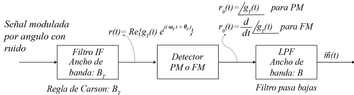
Figura 3.8: Receptor para señales moduladas por ángulo.
