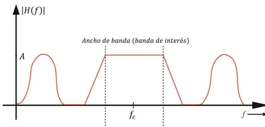
Figura 1. 9: Espectro de un canal pasabanda sin distorsión.
