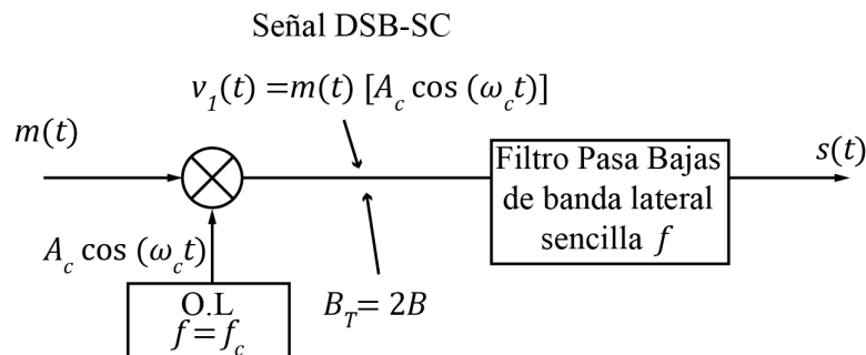
Figura 2.18: Diagrama de bloques para generar SSB por método de filtrado
