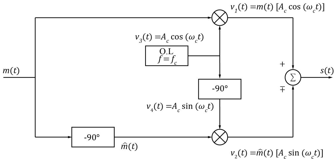
Figura 2.17: Diagrama de bloques para generar SSB por método de fase
