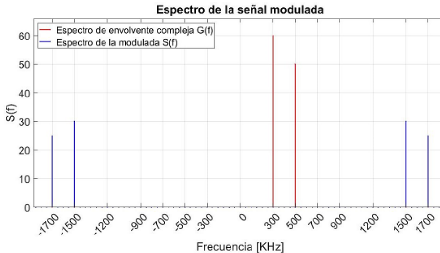
Figura 2.21: Espectro de la envoltura compleja, y señal USSB resultante del ejemplo 2.3.
