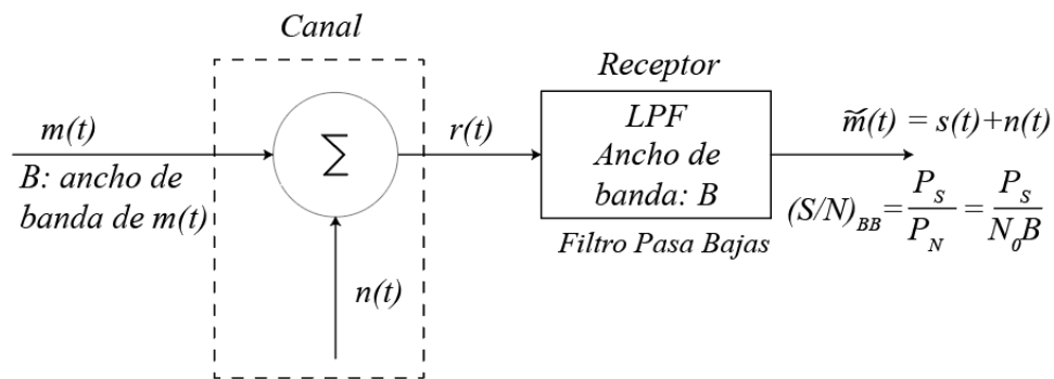
Figura 3.2: Sistema de comunicación banda base.
