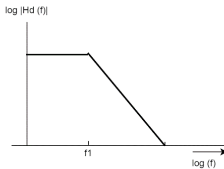
Figura 3.23: Gráfico de Bode de la característica de Deénfasis
