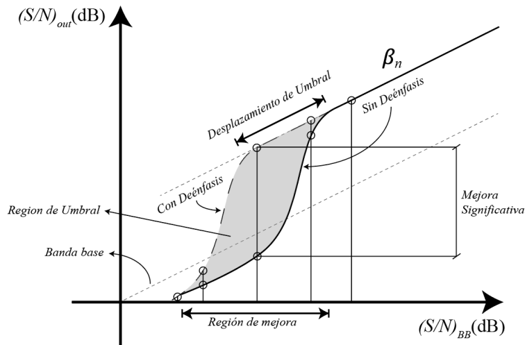
Figura 3.14: Comparativa de rendimiento del ruido de un discriminador de FM para una señal senoidal FM modulada con ruido gaussiano con deénfasis y sin deénfasis.
