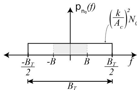
Figura 3.11: DSP para el ruido a la salida del detector para el receptor de señal modulada en PM.
