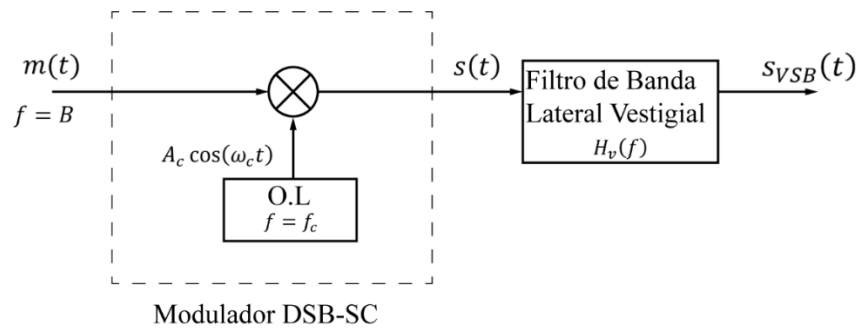
Figura 2.22: Diagrama de bloques de generación de una señal VSB
