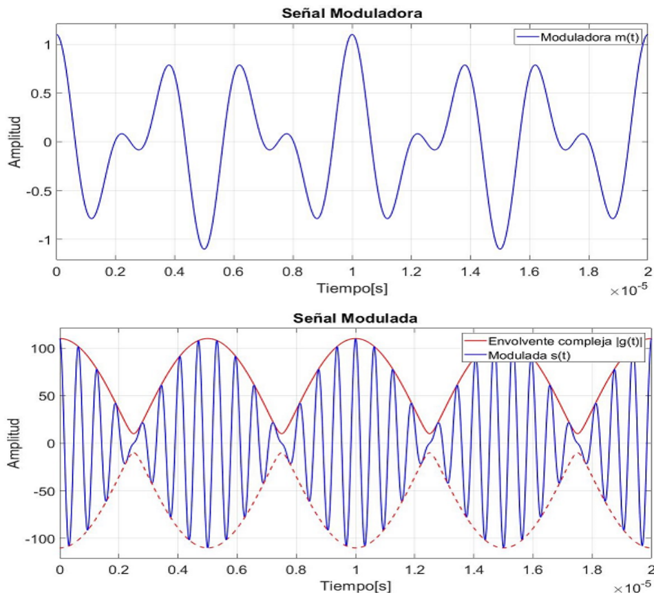
Figura 2.19: Forma de onda de la señal moduladora, señal de la envolvente compleja y señal USB resultante del ejemplo 2.3.
