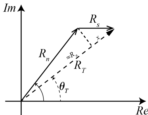
Figura 3.6: Diagrama fasorial de la aproximación de AM.
