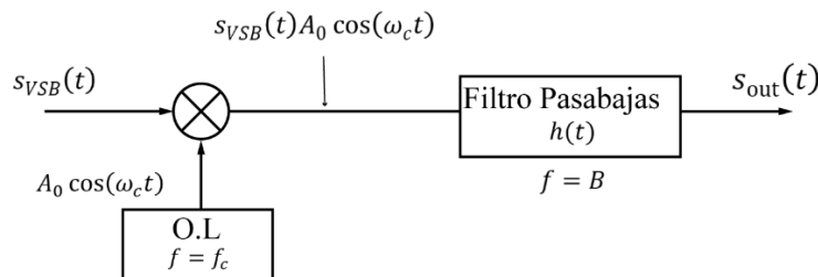
Figura 2.24: Diagrama de bloques de la demodulación VSB por detector de producto
