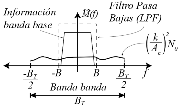
Figura 3.12: DSP de ruido en sistema banda base.
