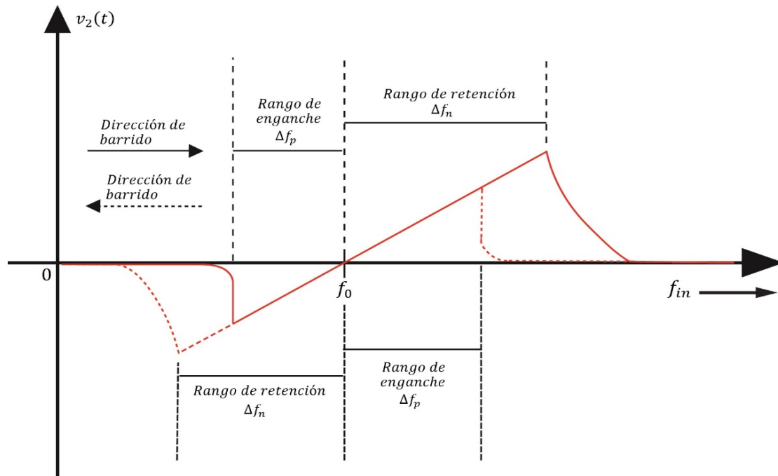
Figura 1. 32: Voltaje de control para el VCO de PLL para un barrido de una señal senoidal de entrada.
