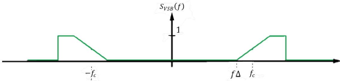
(d) Señal resultante VSB
