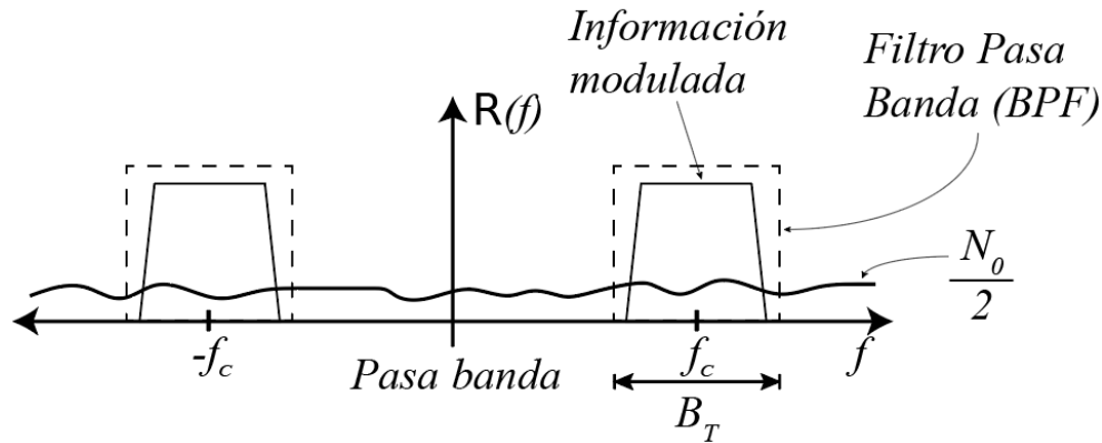
Figura 3.10: DSP de ruido en sistema pasa banda.
