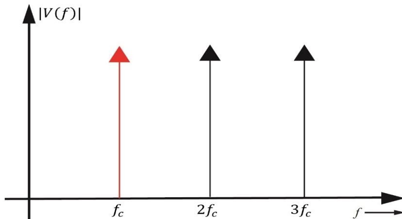
Figura 1. 16: Efecto de la distorsión armónica.
