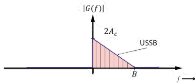
Figura 2.15: Envoltura para modulación SSB.
