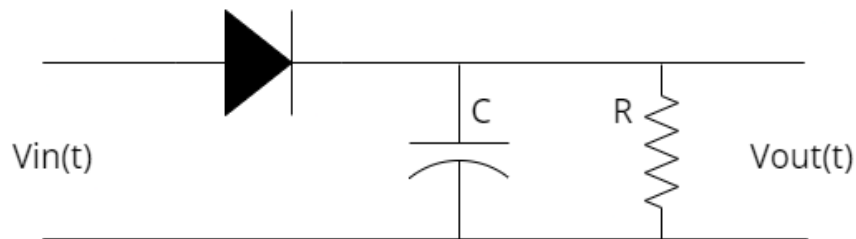
Figura 1. 27: Detector de envolvente con diodo.
