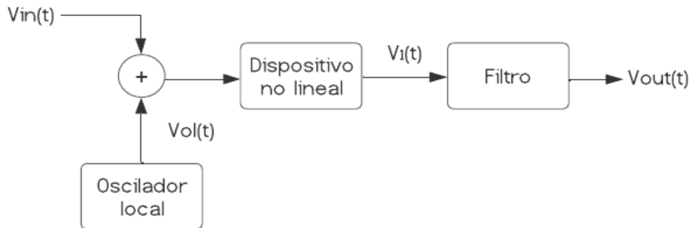
Figura 1. 26: Dispositivo no lineal utilizado como mezclador.
