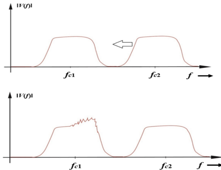
Figura 1. 18: Efecto de la modulación cruzada.
