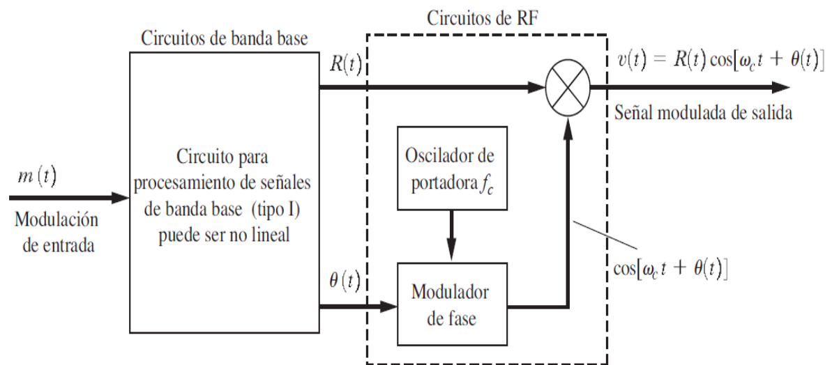
Figura 1. 33: Transmisor generalizado utilizando técnica de generación.
